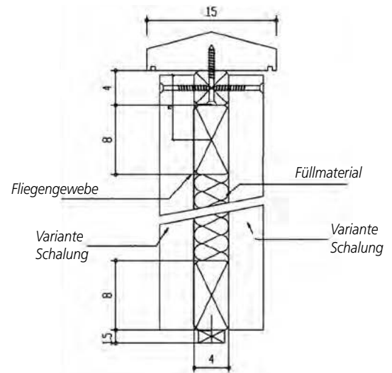
Schallabsorbierende Seite
